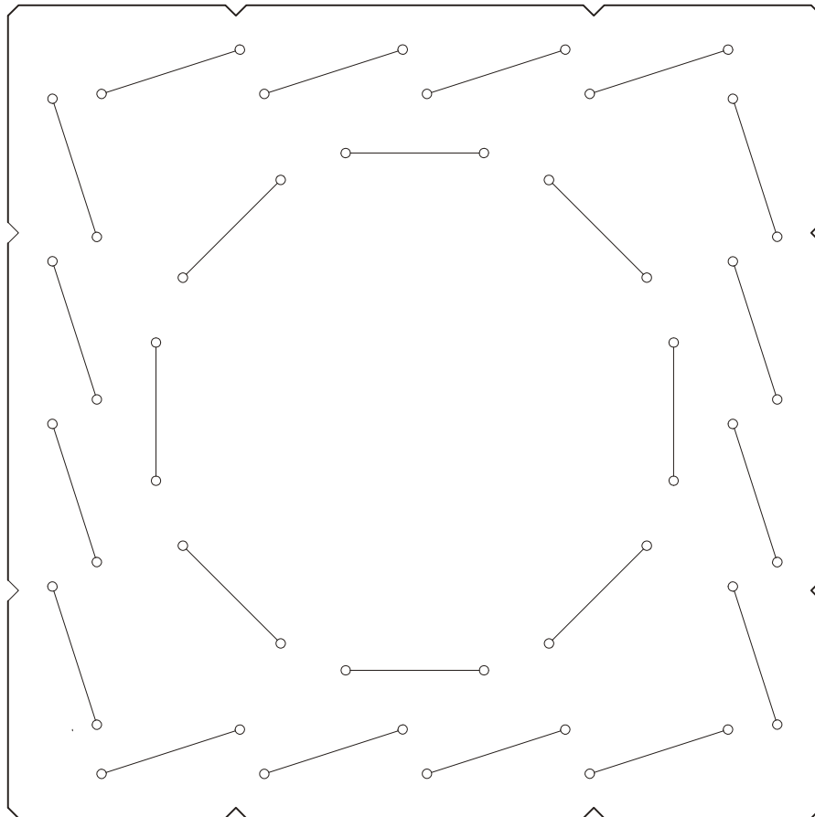
1:1 - Vorlage Flechtschablone
